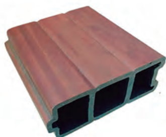
PERFIL DIVISÓRIA 180x73mm PESO: 5,1 Kg/m
